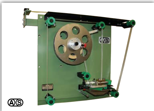
Folienbeleimvorrichtung ohne Trockenstrecke
