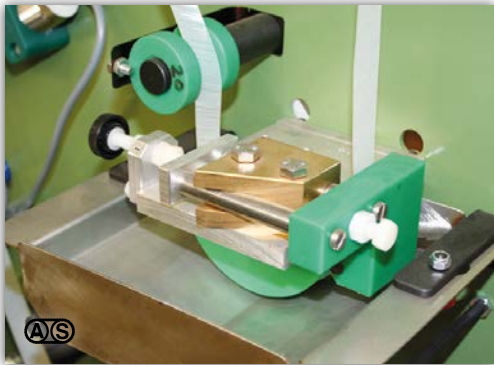
Folienbeleimvorrichtung mit Leimbehälter
