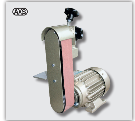
AS-5 Tischmodell, mit beidseitig freiem Arm AS-5 Modèle d'établi, au bras accessible des deux côtés
